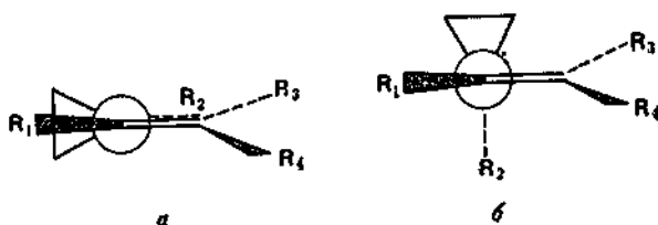
Рис. 4.6. Конформации \alpha -циклопропилалкенов. В конформации a сопряжение максимально, в конформации б — минимально.
