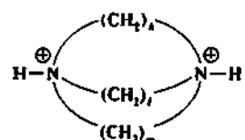
изомер «наружу-наружу»
