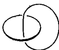
[2] катенан
