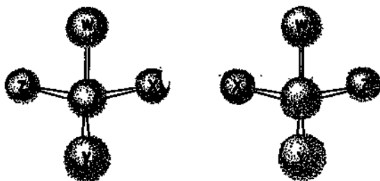
Рис. 4.1. Энантимеры.
