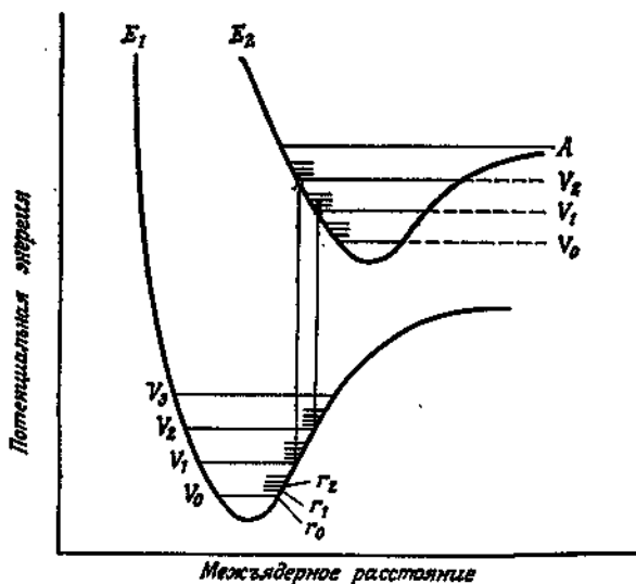
Рис. 7.2. Диаграммы энергии двухатомной молекулы. Показаны два возможных перехода. Если электрон возбужден до уровня А, молекула может распасться (разд. 7.5).
