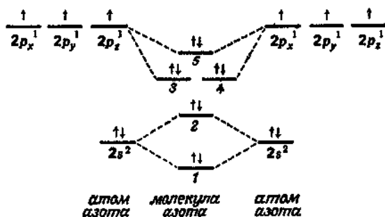
Рис. 1.9. Электронная структура молекулы азота N_2 (электроны внутренней оболочки не показаны) [12].
