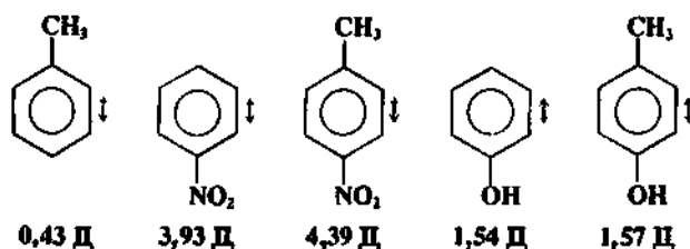
Рис. 1.10. Величины дипольных моментов (Д), измеренные для некоторых производных бензола. Стрелка указывает на более электроотрицательную часть молекулы [29].
