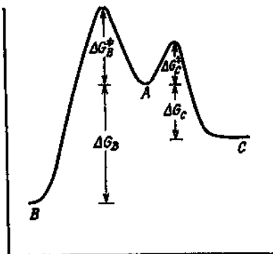
Рис. 6.3. Диаграмма свободной энергии реакции, иллюстрирующая кинетический и термодинамический контроль продукта. Исходный реагент А может давать или продукт В, или продукт С.
